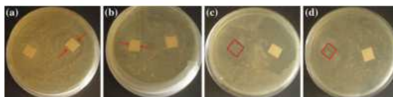
شکل 5 نتیجه آزمون فعالیت ضد باکتریایی ، a فیلم ۱۰ لایه nano-ZnO ، b پارچه های فیلم رسوب یافته ZnO
