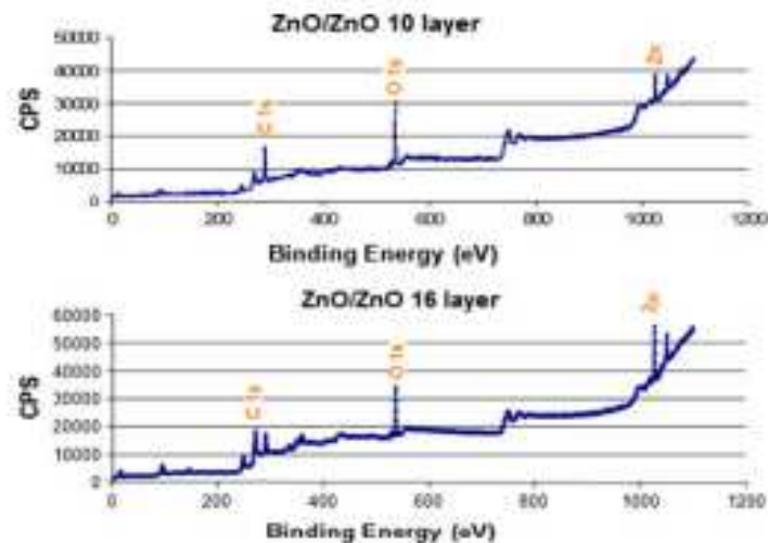
شکل 2 طیف XPS از ۱۰ و ۱۶ فیلم چندلایه nano-ZnO رسوب یافته در پارچه پنبه ای بافته شده باردار مثبت
