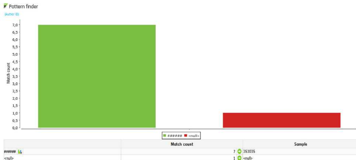
شکل ۸. یابنده الگو
