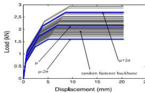
(d) ductile random fastener backbone model
