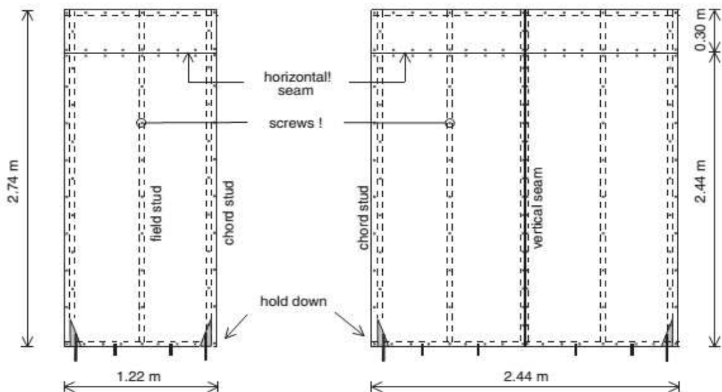
شکل 4: پیکربندی دو دیواره ی برشی، ارائه شده توسط لیو و همکاران برای آزمایش دیواره های برشی CFS: 1/22
