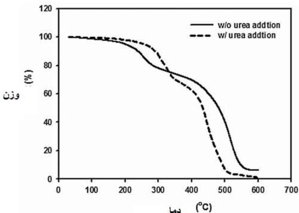
شکل 5: منحنی کاهش وزن TGA میکرو کپسول های پلی اورتان و میکرو کپسول های PUF رسوب دهی شده با UF
