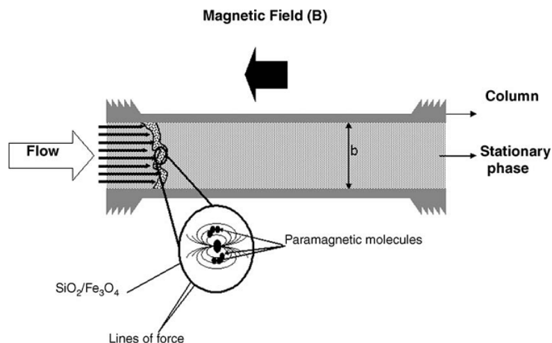
عکس. 1. ویژگی‌های ستون کروماتوگرافی
