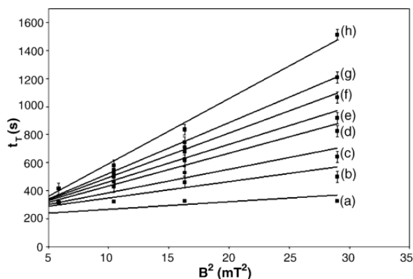
شکل 6 نمودار t_r (s) در برابر مربع میدان مغناطیسی ( \text{mT}^2 ).
