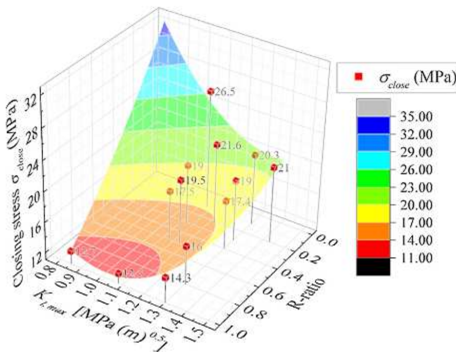
شکل 13: نوسانات تنش بستار با K_{1,max} و نسبت R در فرکانس 1 هرتز.
