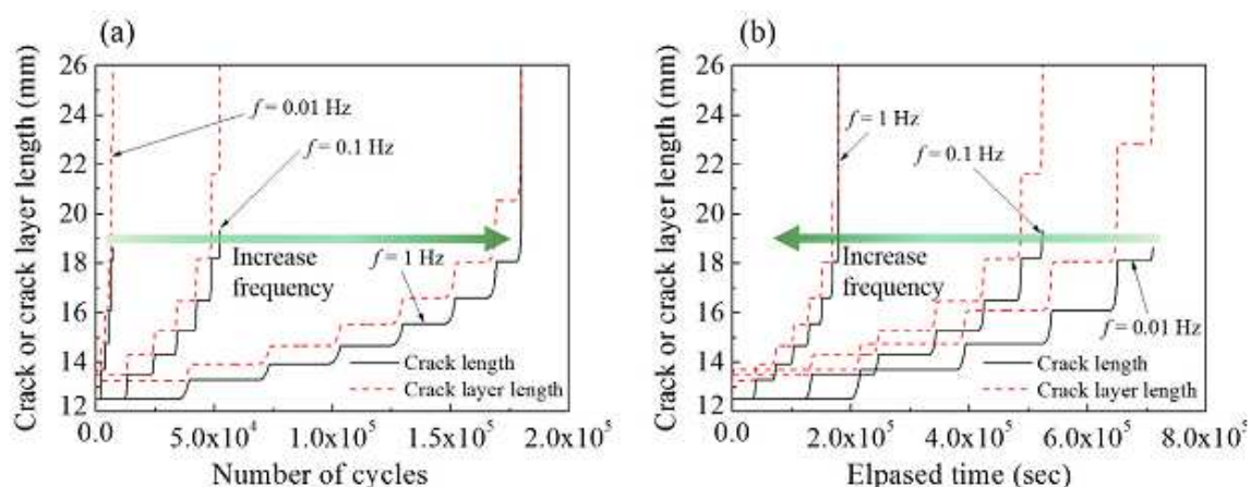
شکل 8: ترک و انشار لایه ترک در فرکانس های خستگی مختلف ( f = 1, 0.1, 0.01 Hz)، (a) طول ترک و لایه ترک با تعداد سیکل ها و (b) طول ترک و لایه ی ترک با زمان
