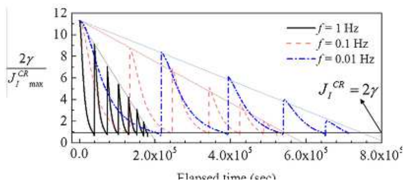
شکل 9: تغییر انرژی شکست سطحی نرمال شده با نرخ انرژی آزاد شده در راس ترک در فرکانس های مختلف
