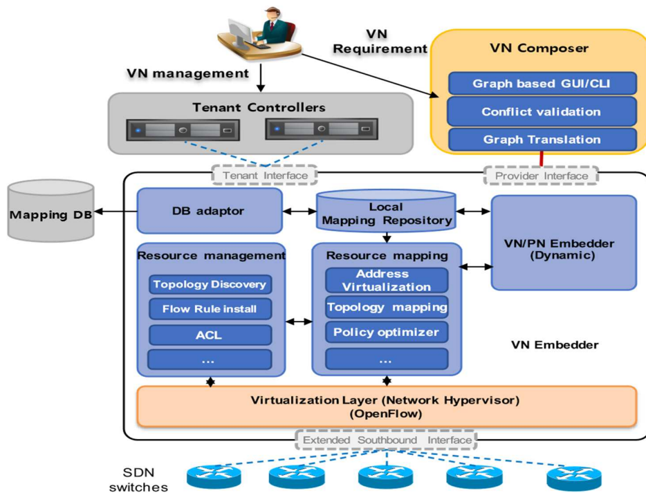
شکل 1- معماری کلی
