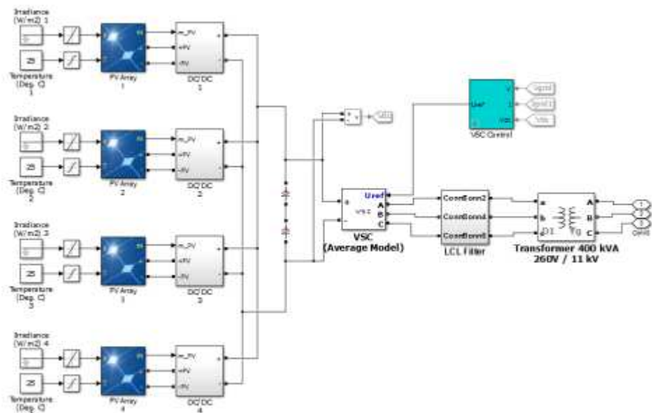
شکل 2: زیر سیستم فتوولتائیک
