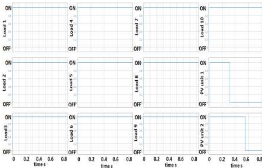
شکل 11: نمودار وضعیت مدار شکن در طی سناریو 2
