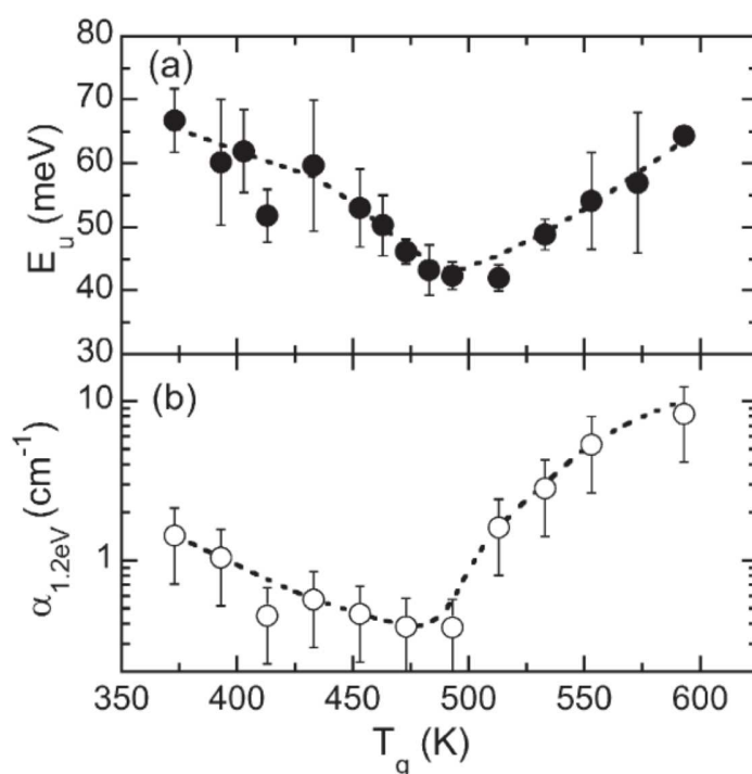
شکل 7. (a) انرژی Urbach, E_u , (b) ضریب جذب در 1.2 الکترون ولت، \alpha_{1.2eV} ، به عنوان تابعی از T_g , E_u در گستره \approx 40 \text{ meV} تا \approx 65 \text{ meV} است و حول و حوش T_g = 493 \text{ K} مینیمم می شود. (b) \alpha_{1.2eV} در گستره \approx 0.3 \text{ cm}^{-1} تا \approx 10 \text{ cm}^{-1} برای فیلم های a\text{-Si:H} رشدیافته در T_g = 373 \text{ K} تا 593 \text{ K} است. خطوط نقطه نقطه، راهنماهایی برای چشمان هستند.
