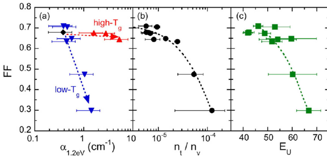
شکل 10. FF به ازای \alpha_{1.2\text{eV}} ، n_t/n_v و E_U . (a) FF به شدت وابسته به \alpha_{1.2\text{eV}} ، فقط برای فیلم های
