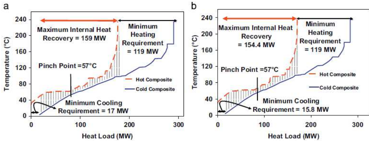
شکل 15: الف) نمودار پینچ دو ب) نمودار پینچ 3. نمودار پینچ 2 بعد از اجرای اصلاح مجدد اب. دیاگرام پینچ 3 بعد از حذف نقاط nim.
