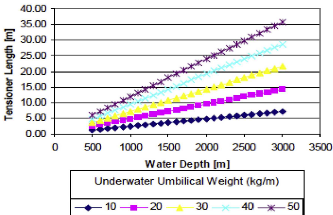
شکل 9: افزایش طول در برابر عمق آب و وزن کابل مرکزی (Dieumegard & Fellows . 2003)
