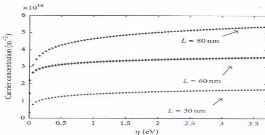
شکل 6: غلظت حامل با توجه به n برای مقادیر مختلف L
