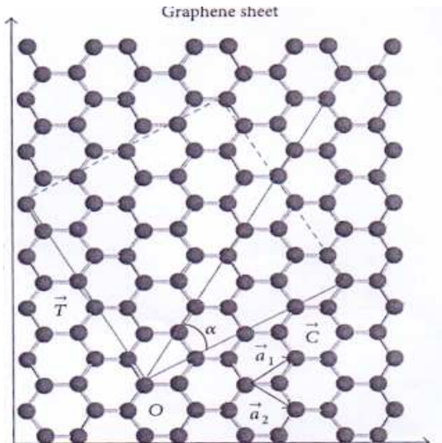
شکل 1: مدل شماتیک نانواسکرول گرافن
