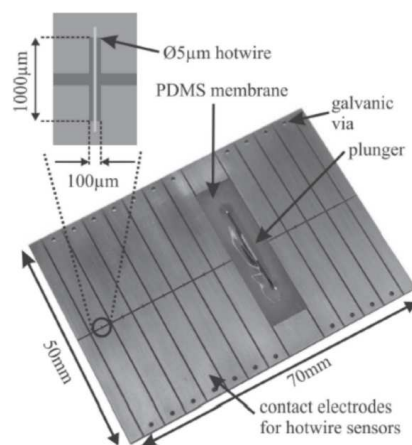
تصویر 6. سیستم کامل برای تاخیر فعال انتقال با PCB، محرک، غشاء و سنسورهای جریان سیم داغ
