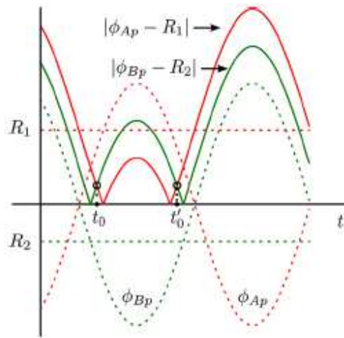
شکل (8). لحظه بسته شدن بهینه که راه حل مسئله مینیمم ماکزیمم است
